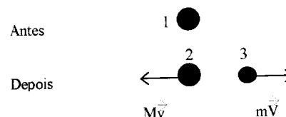
Figura 8: A conservação do momentum no decaimento da partícula 1.
