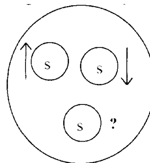
Figura 14: O problema dos spins dos três quarks s no bárion \Omega^- .
